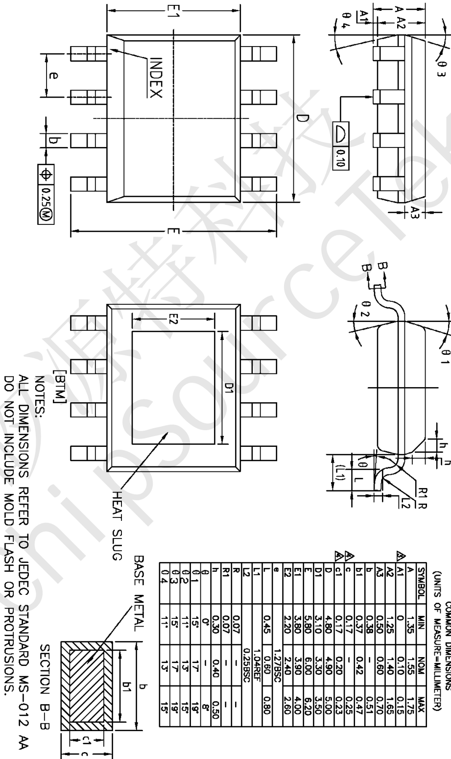
AXS2031封装图 (ESOP8)
