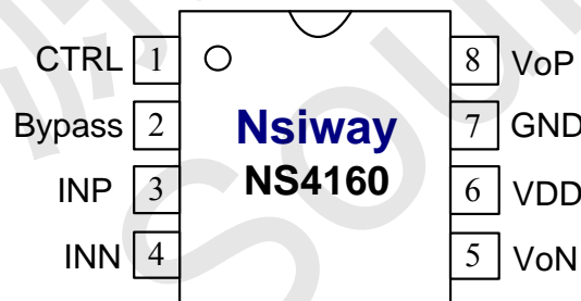
图2 SOP8 装管脚分配图(top view)
