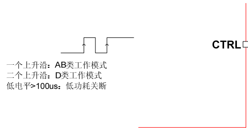
图4 NS4163 工作模式设置
