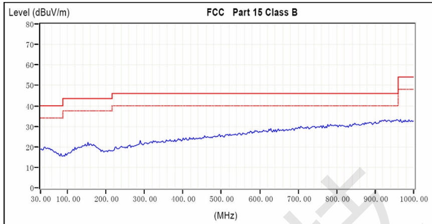
图4 EMI 测试频谱图
