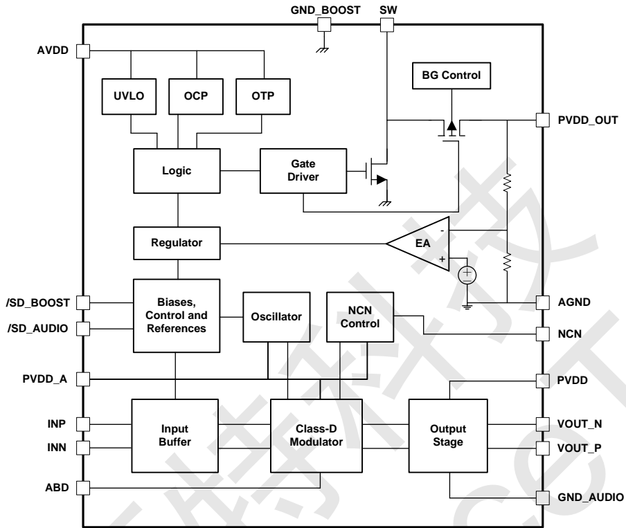
图3 NS4752 原理框图
