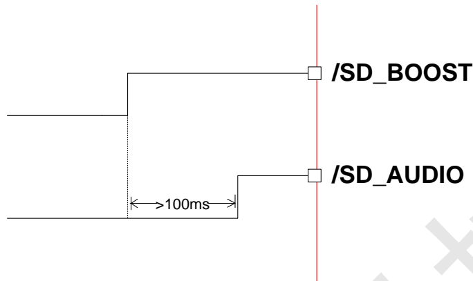
图7 NS4752 软启动时序
