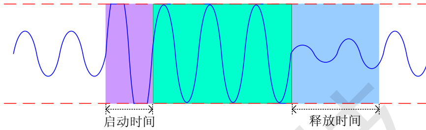
图5 普通工作模式下的音频输出信号
